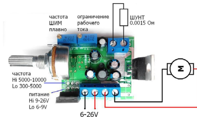
Эскиз подключения
